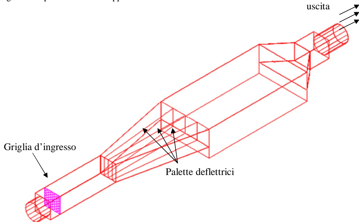
Figura 5. Esempio di vista tridimensionale di una wind tunnel
